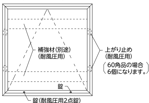
(真下からの図)
