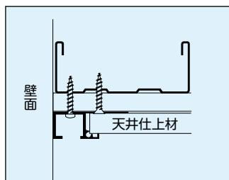
施工例1<天井付け>
