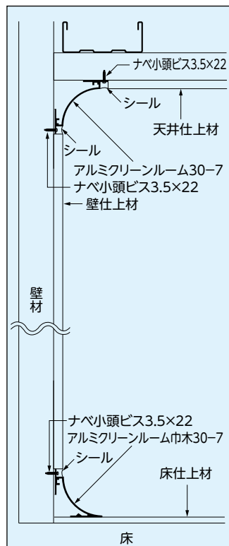
施工例・断面図
