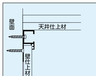
施工例2<壁付け>
