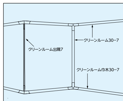
施工例・全体図1
